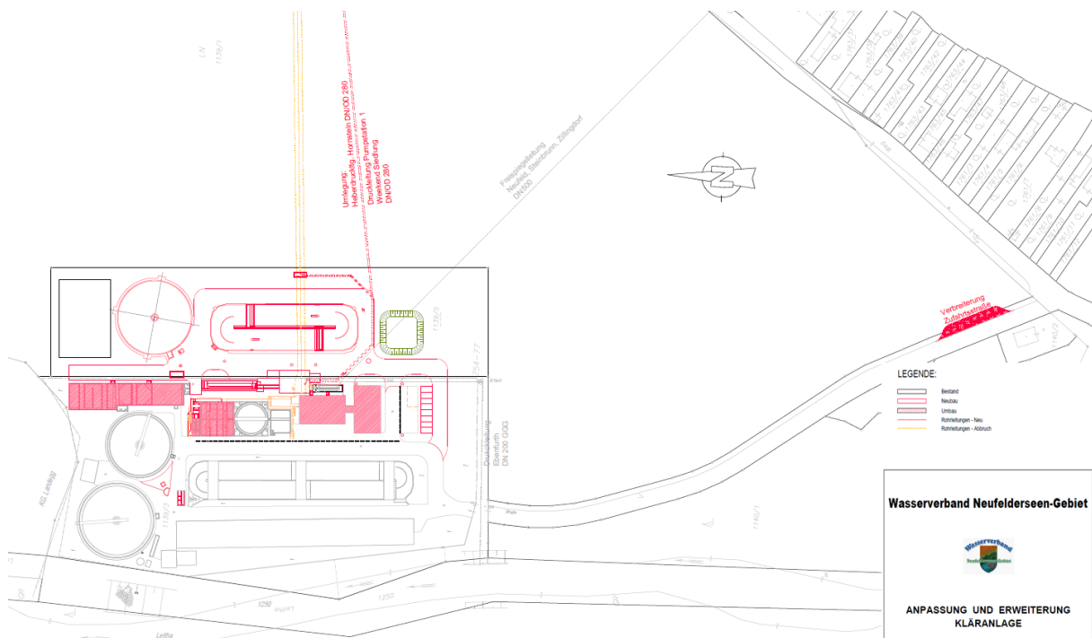
Bild: Auszug Lageplan Baumaßnahmen Kläranlage (BA18)
